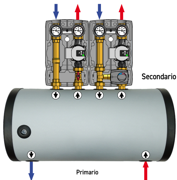
Schema di applicazione: volano termico montaggio orizzontale
