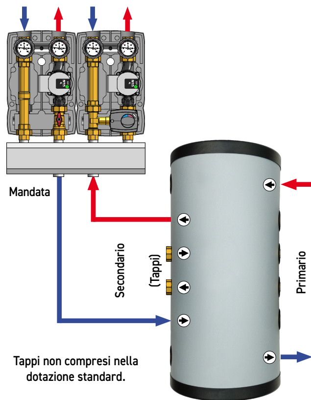
Schema di applicazione: volano termico montaggio verticale
