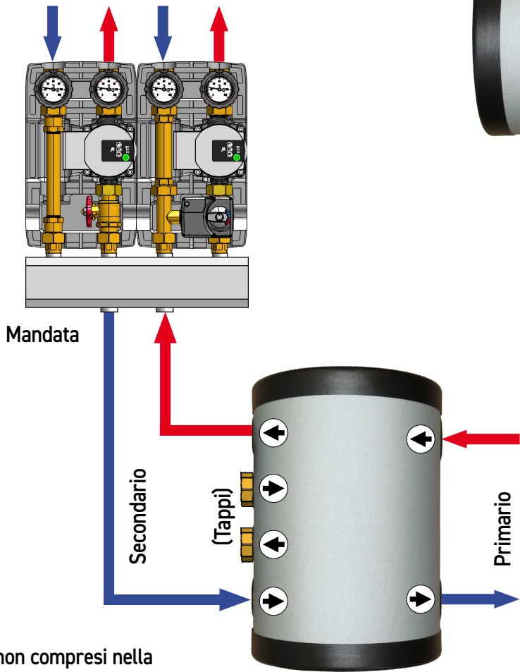
Schema di applicazione: volano termico montaggio verticale
