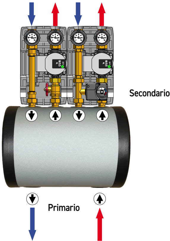
Schema di applicazione: volano termico montaggio orizzontale
